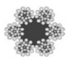
6x26WS
