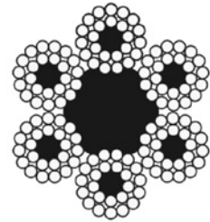
6x24
