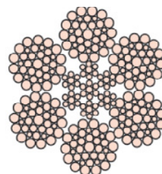
Hyflex 6
