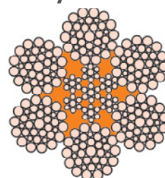
Hyflex 6P
