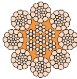
Hyflex 8P
