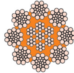
Hyflex 8x19P
